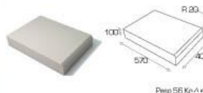
Peça lateral (dreta o esquerra)
